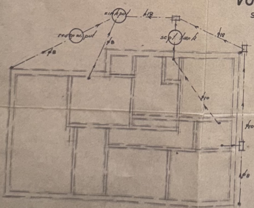
fundering schaal 1/100
