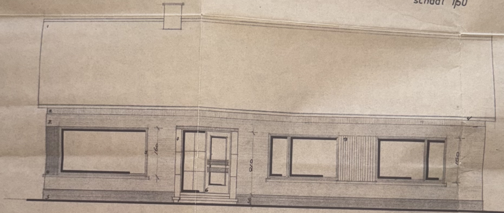
voorgevel schaal 1/50
