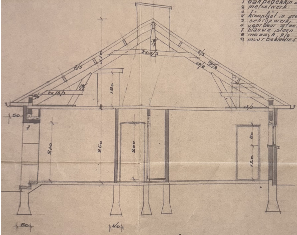
snede a-a schaal 1/50
